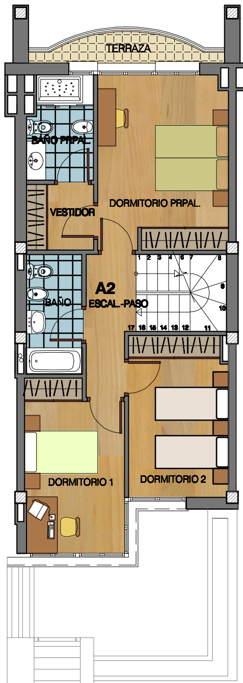
PLANTA PRIMERA
